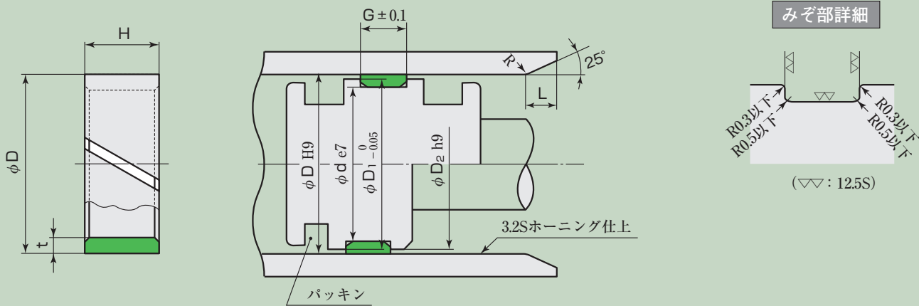
SWウェアリング寸法表
